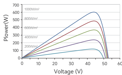
Power-Voltage(600W)
